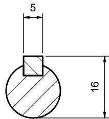
A-A ( 1 : 1 )
