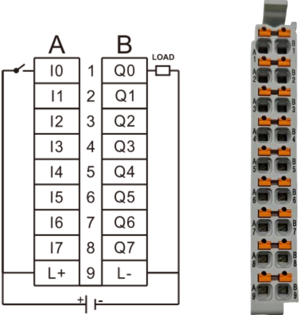
Fig.7.4-1 RP20-0808DTP wiring diagram
