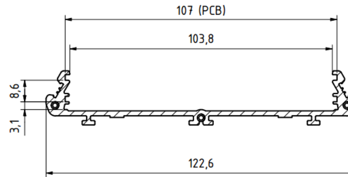
A-A ( 1 : 1 )
